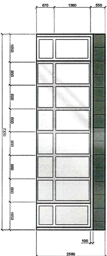
ФАСАД
