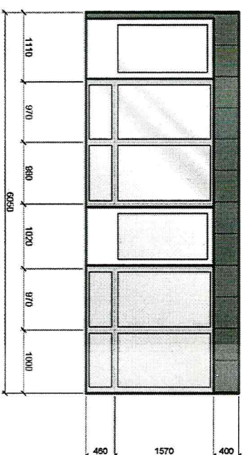
ФАСАД
