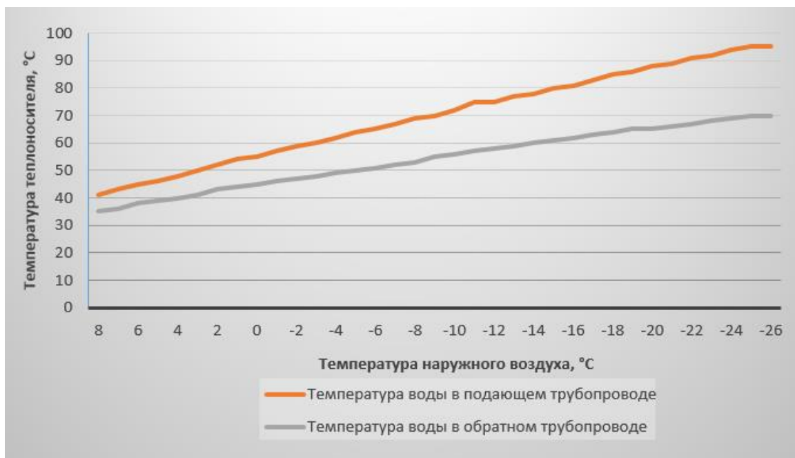
Рисунок 5.8.1.– График изменения температур теплоносителя 95–70 °С.
