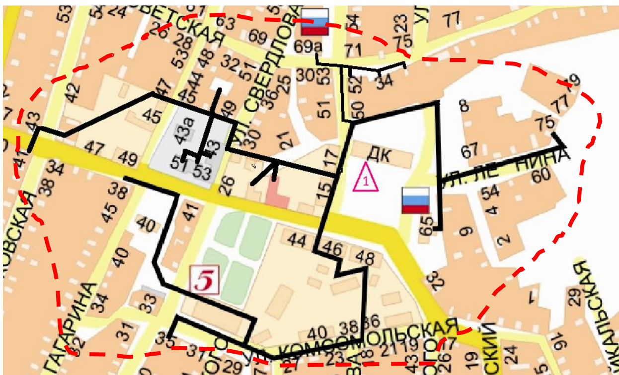
Рисунок 2.1.1 - Зона действия котельной №1.
