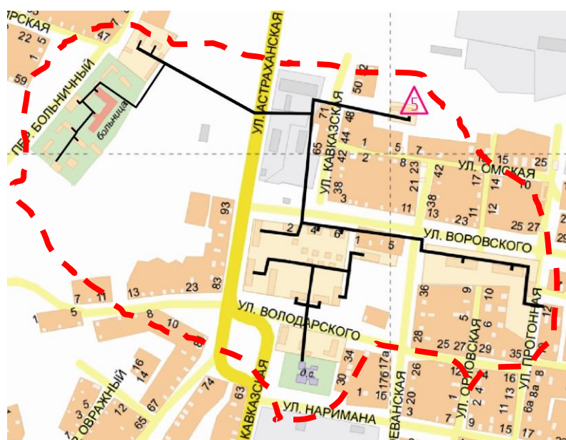
Рисунок 2.1.3 - Зона действия котельной №5.
