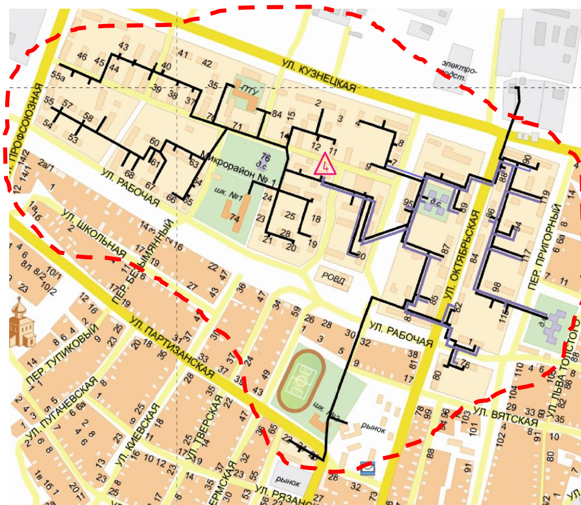
Рисунок 2.1.2 - Зона действия котельной №4.
